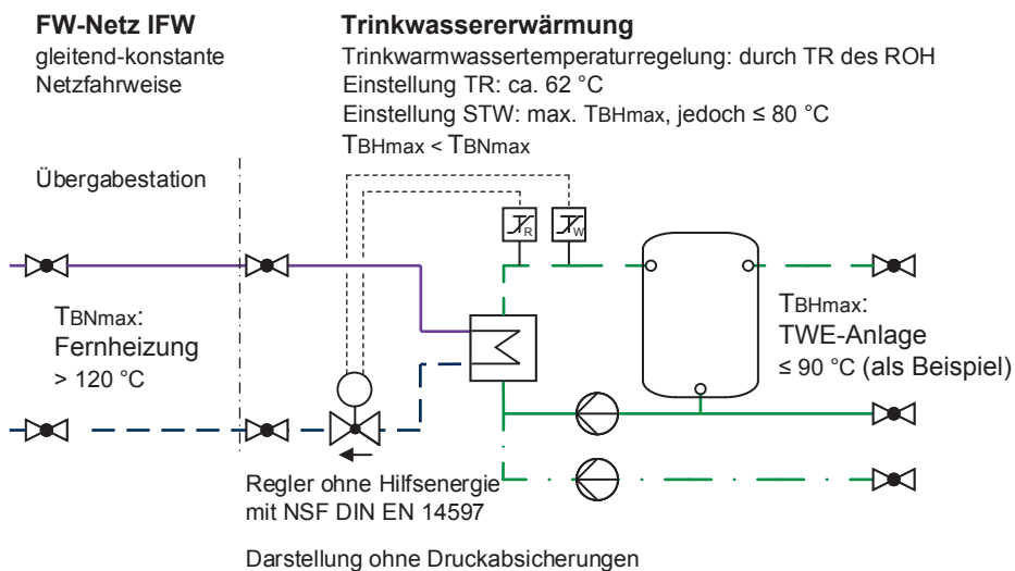
Bild 2: Erforderliche sicherheitstechnische Temperaturabsicherung gemäß Kapitel 8.1.2 bei Verwendung von Reglern ohne Hilfsenergie
