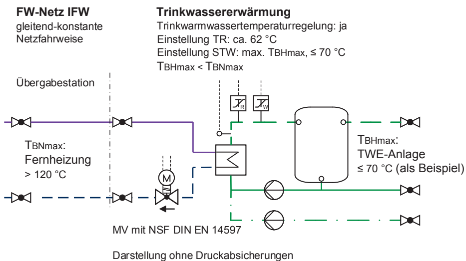
Bild 3: Erforderliche sicherheitstechnische Temperaturabsicherung gemäß Kapitel 8.1.2 bei Verwendung von elektrischen Reglern
